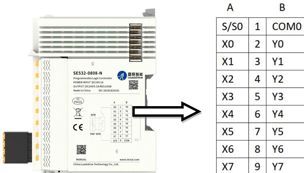
图4-1 产品右侧端子丝印示图
