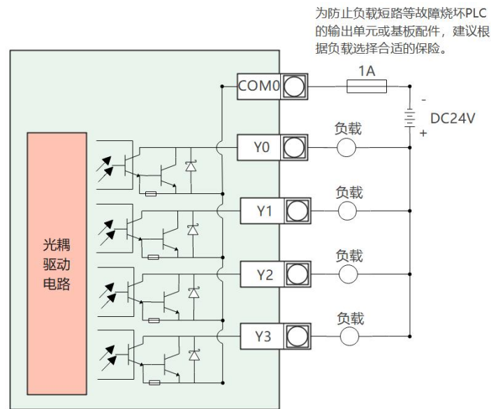
图3-3 普通晶体管输出接线图
