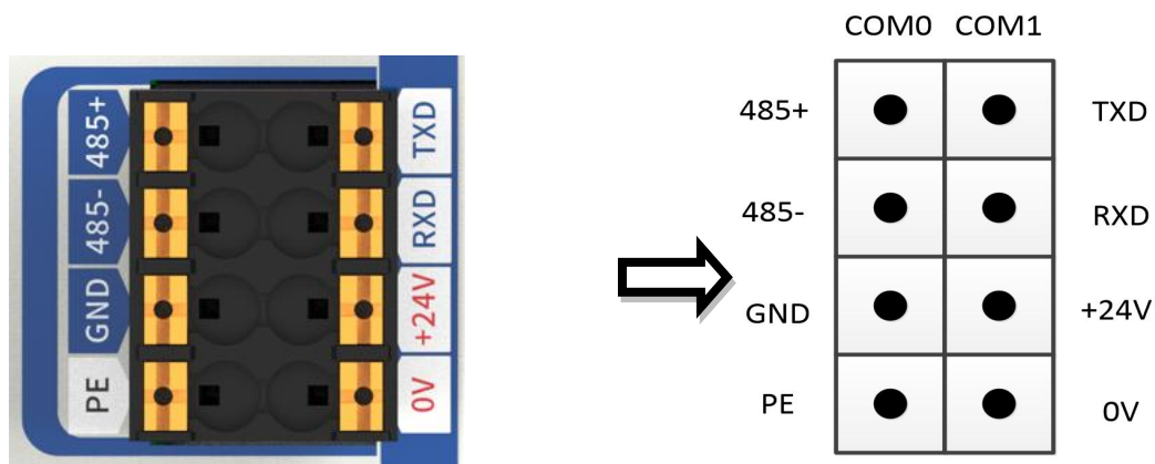
图5-3 RS485&RS232通信端口示意图
