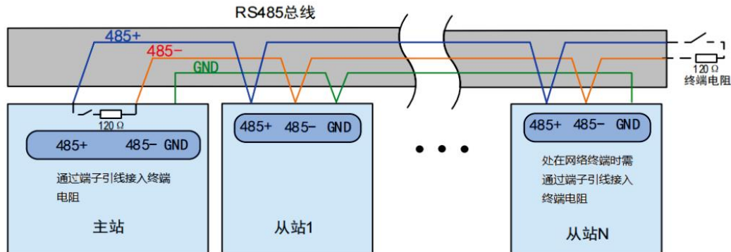
图5-4 RS485总线通信示意图
