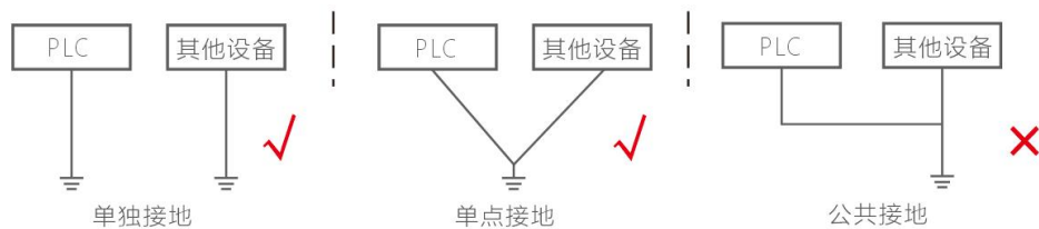
图 1-1 接地类型图
