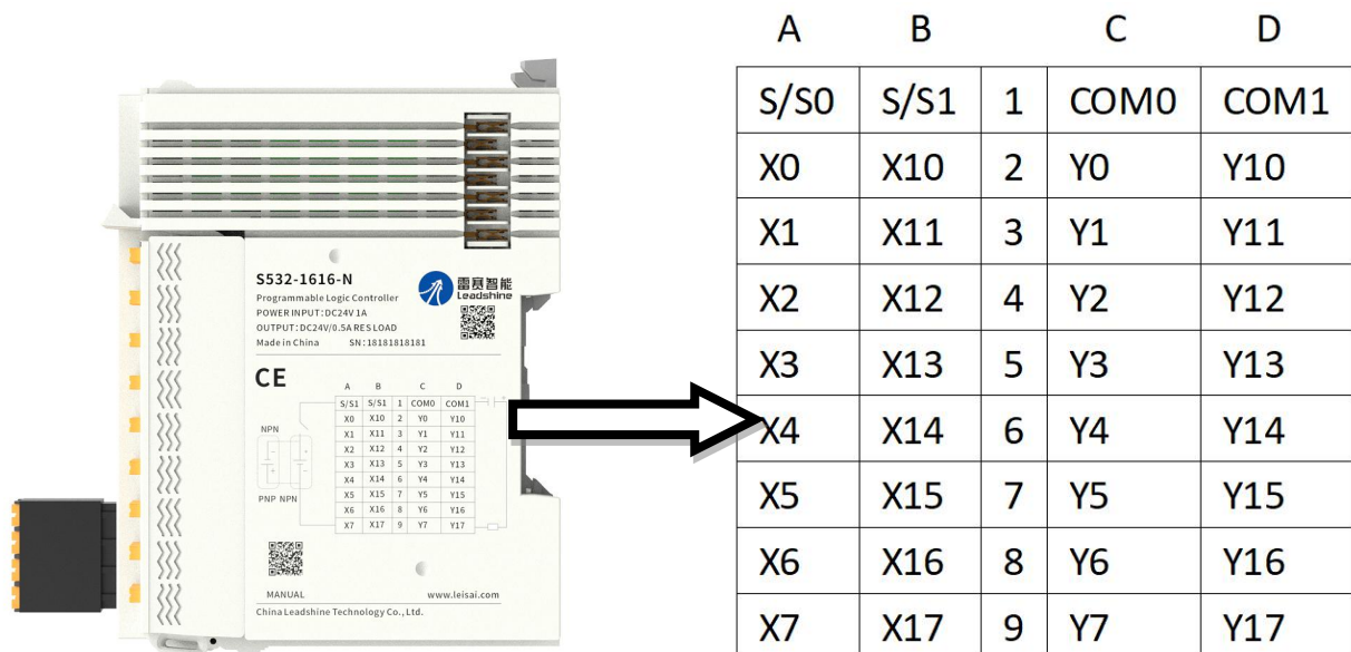
图4-2 产品右侧端子丝印示图
