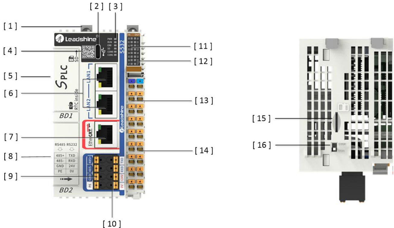
图2-1 S5系列16点IO产品正面外部接口图
