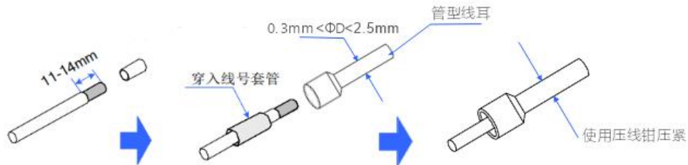
图 4-6 线缆制作示意图
