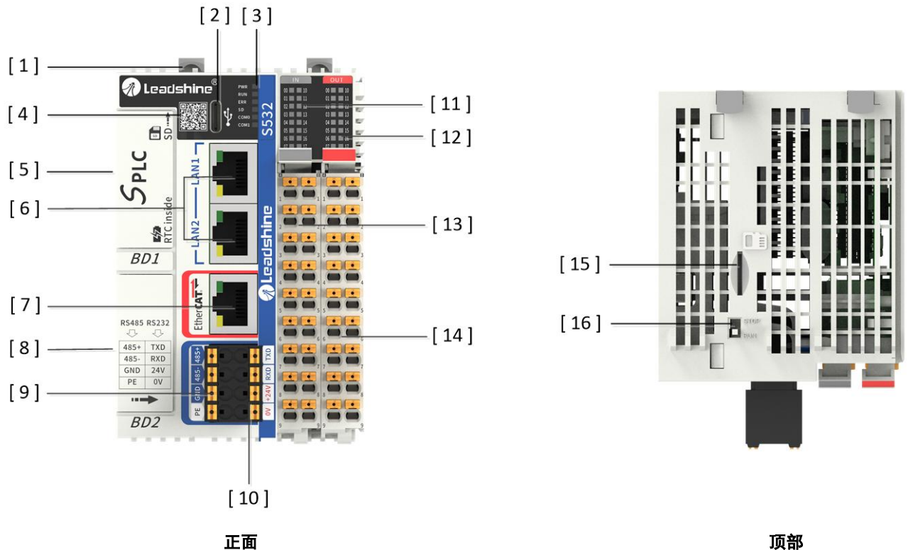
图2-2 S5系列32点IO产品正面外部接口图
