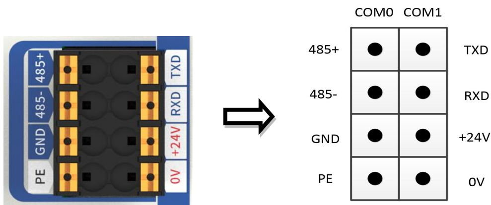
图4-3 电源&通讯端子引脚图
