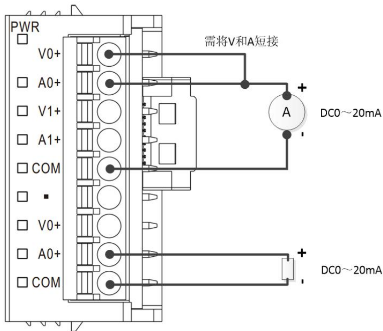
图6-2 S-2AD1DA-VI-BD扩展板接线示意图
